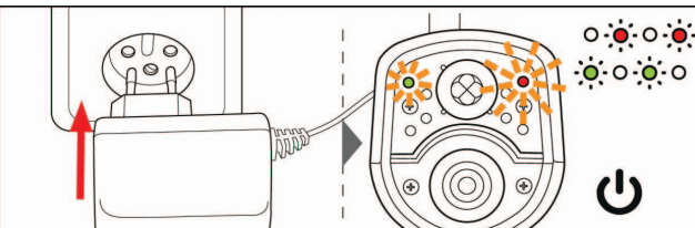
Вставьте адаптер питания в розетку. Камера автоматически включится. Подождите 30 секунд и проверьте светодиоды на передней панели камеры EYE-02.
