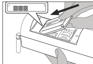
Вставьте аккумулятор и затяните винты.
